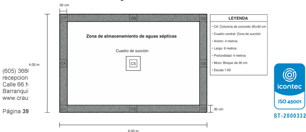
Plano Arquitectónico – Pozo Séptico Dragon Tubulars - Malambo
