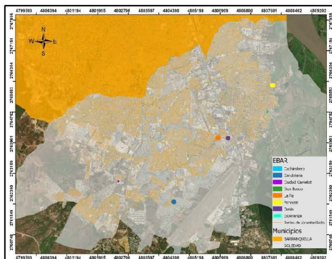
FIGURA 1. REDES DE ALCANTARILLADO INSTALADAS. FUENTE: TRIPLE A DE B/Q S.A. E.S.P.
